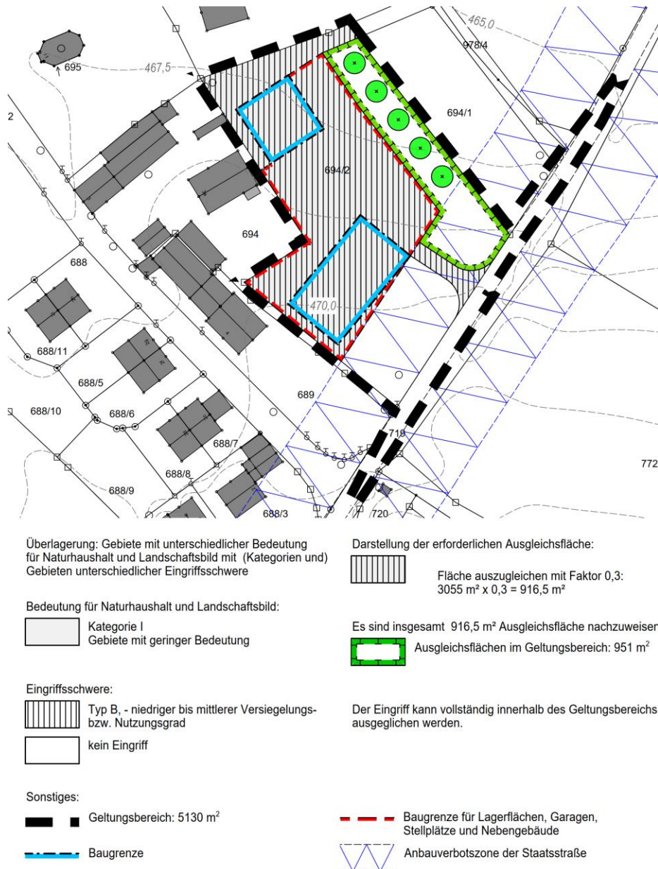
Abb. 4: Plandarstellung der Eingriffsflächen unmaßstäblich, Eingriffsflächen grau hinterlegt, schwarz schraffiert, grüne T-Linie – Ausgleichsflächennachweis, inkl. Zeichenerklärung und Berechnung zur Eingriffsregelung.
